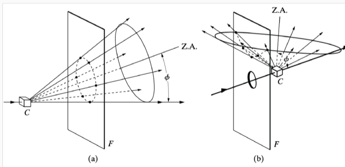
冯-劳厄衍射: (左) 透射和 (右) 反射
