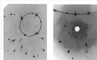
单晶衍射图样
