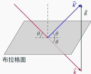
布拉格面: 倒格矢 \vec{g} 的垂直平分面
